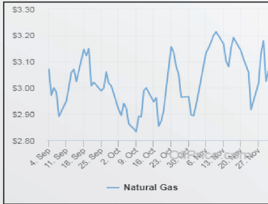
روند قیمت گاز در سه ماه گذشته ($/MMBTU) Oilprice.com
